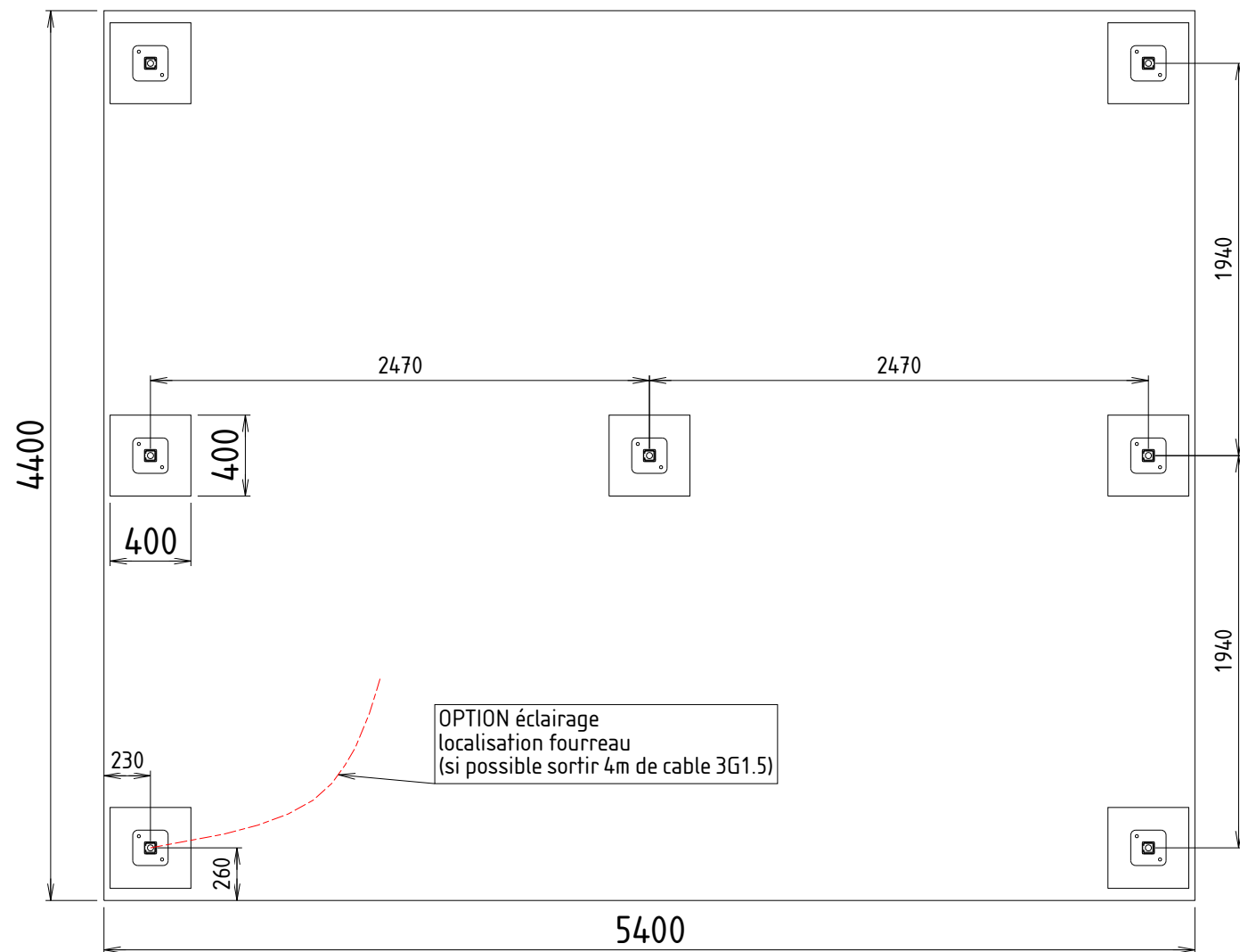
A - A
